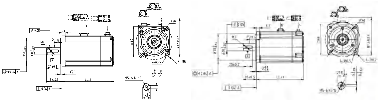
Dimensions
