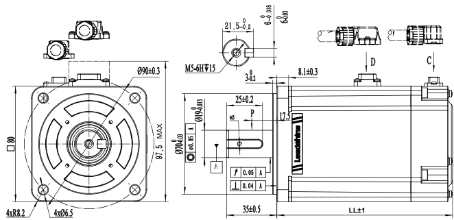
Dimensions
