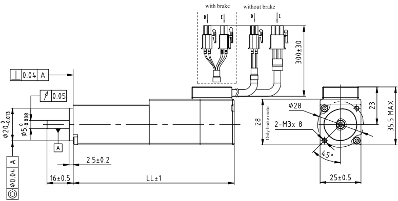
Dimensions
