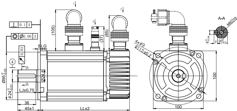
Dimensions
