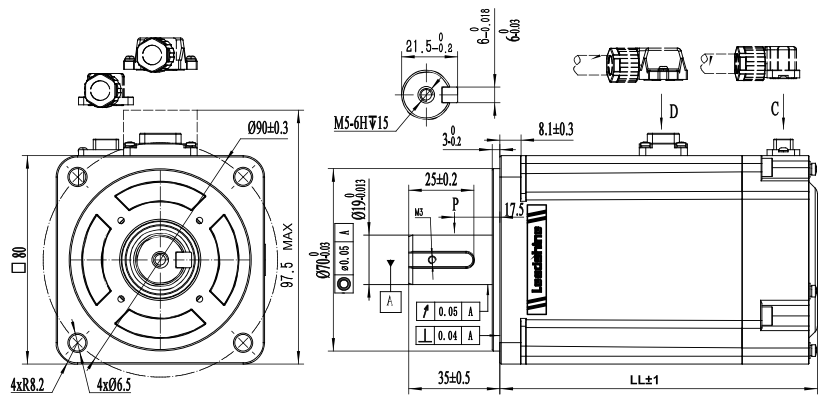
Dimensions
